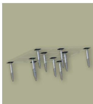
Schraubfundament Berry 1) Schraubfundament enthält die Erdschrauben. Aufnahmen, Befestigungsmaterial und die Einschraubhilfe
